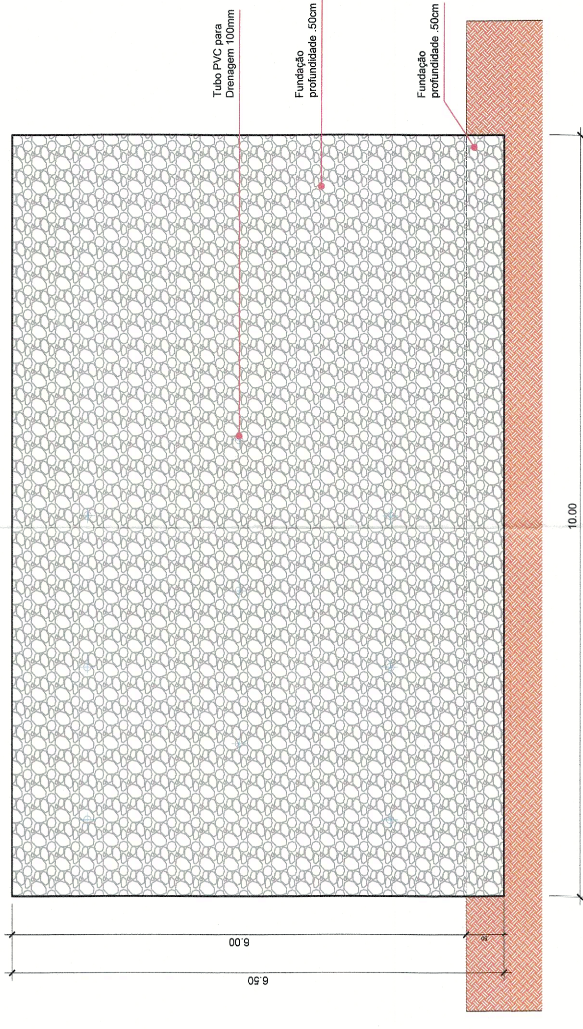
Elevação Frontal Escala: 1/50
