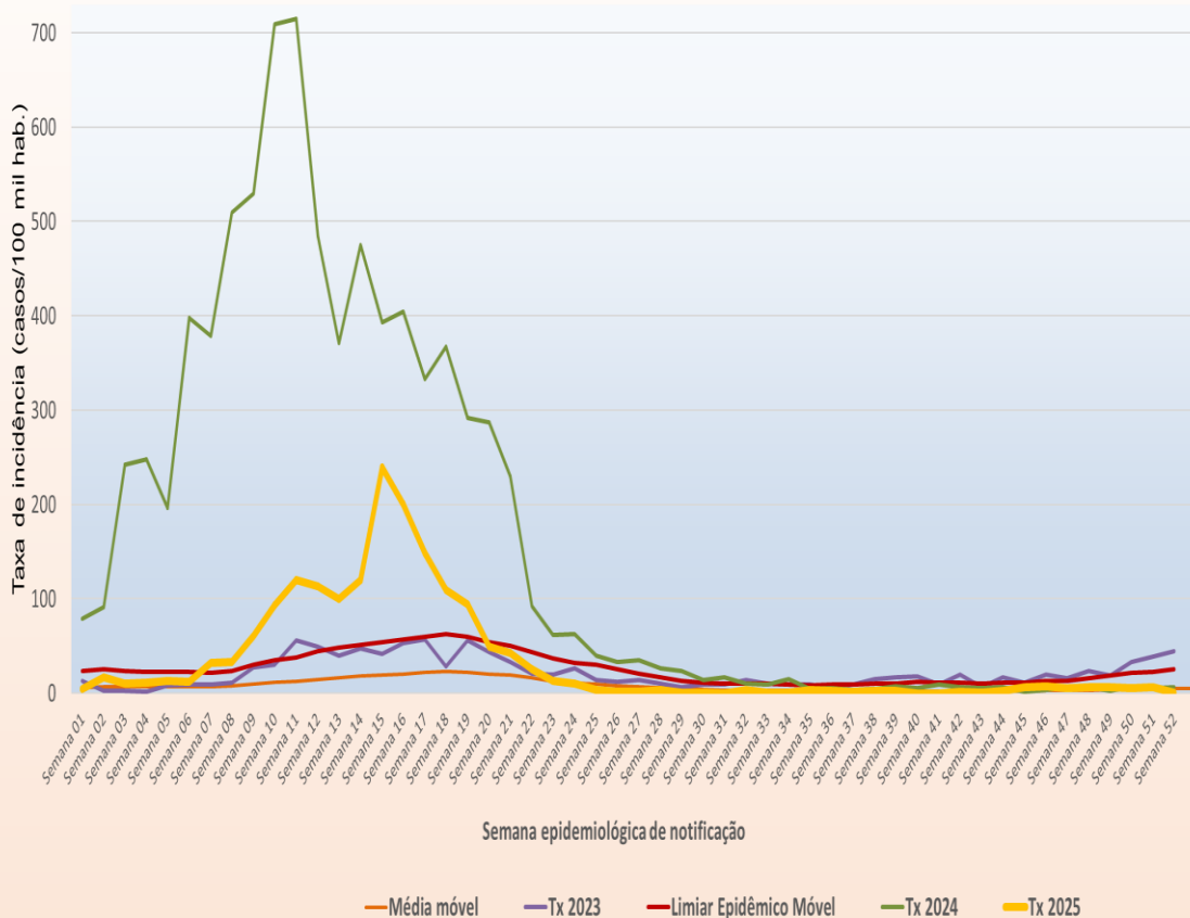
Diagrama de controle da dengue em Angra dos Reis (2024/2025).
