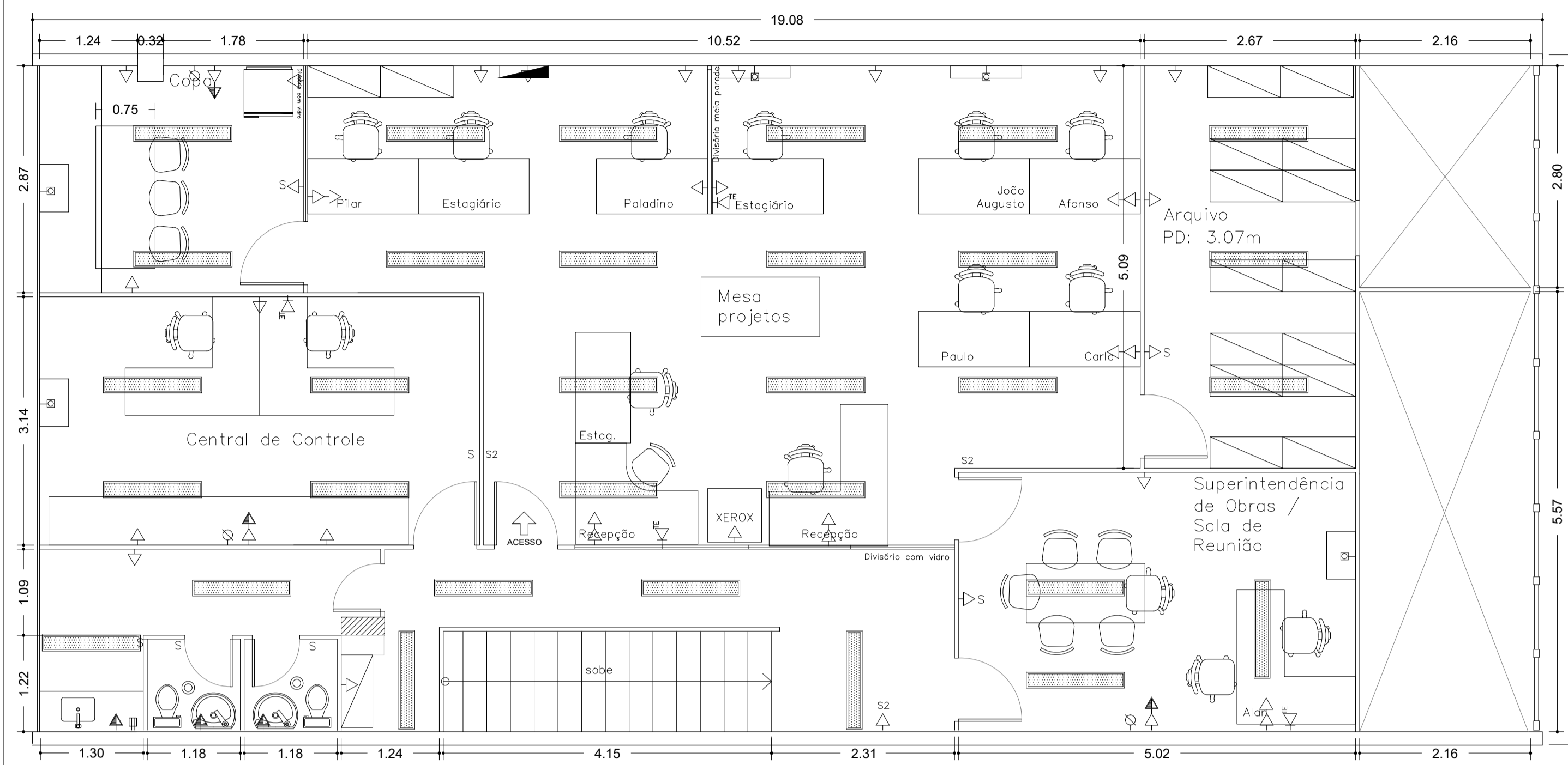
1 PLANTA BAIXA - PRIMEIRO PAVIMENTO Escala: 1/50
