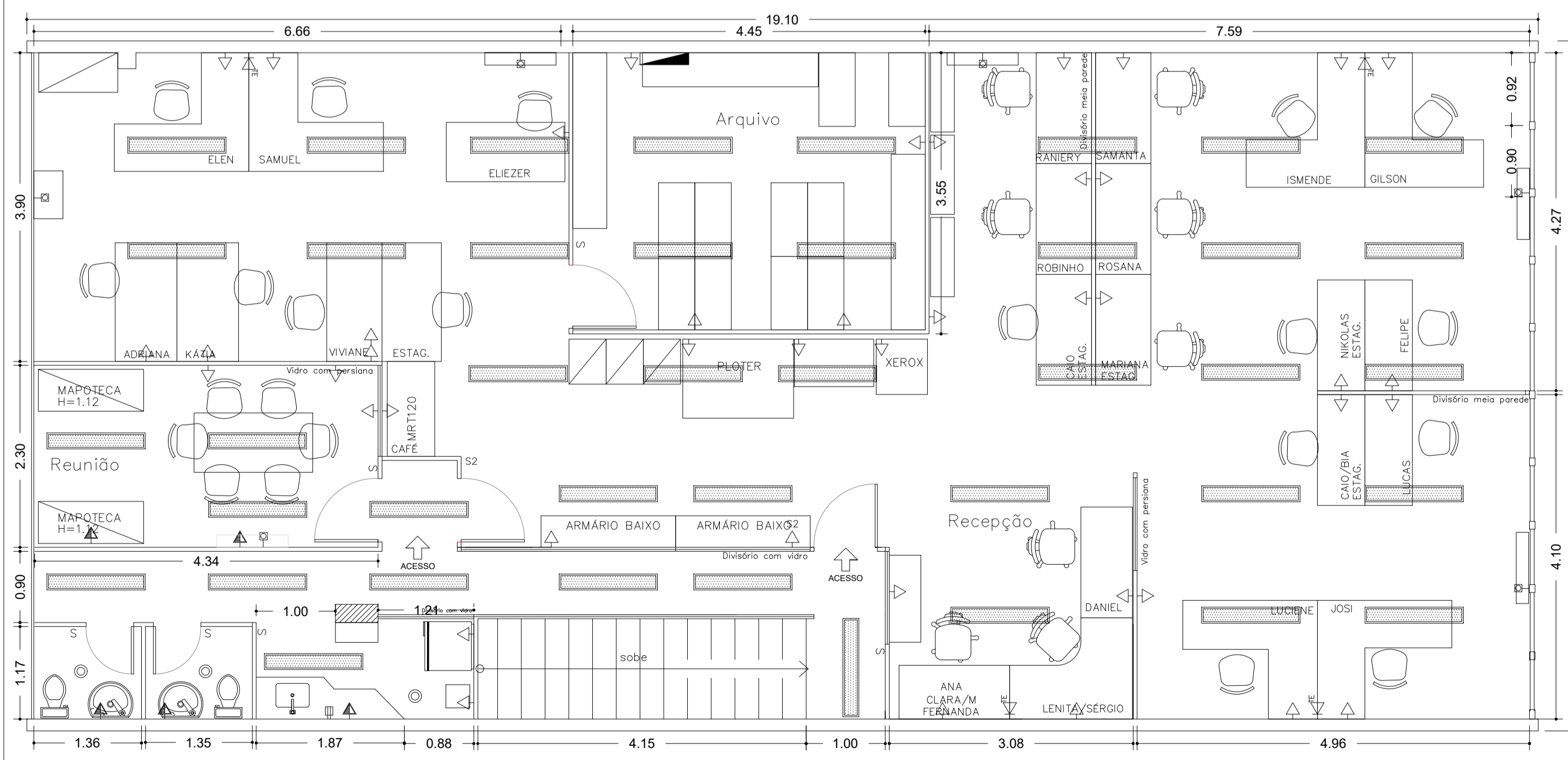
3 PLANTA BAIXA - TERCEIRO PAVIMENTO Escala: 1/50
