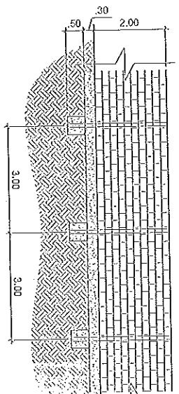
4 Corte Frontal do Muro
